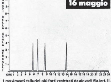
I movimenti tellurici più forti registrati da giovedì 6 a ieri, 15 un'onda (tratteggiata) ha avuto per epicentro Lubiana.
