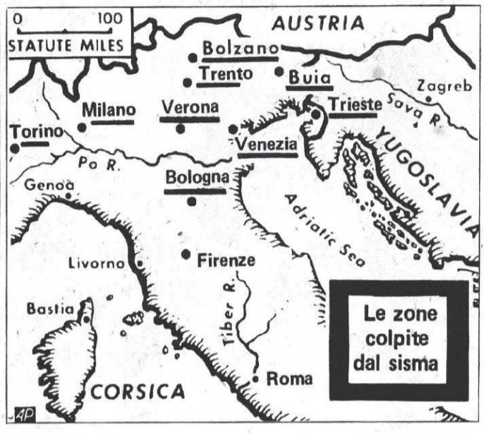
ROMA - La mappa indica le zone dove il sisma ha raggiunto la maggiore intensità. (Tel. Ap)
